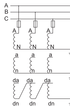
常规接线方式 Routine wiring diagram
